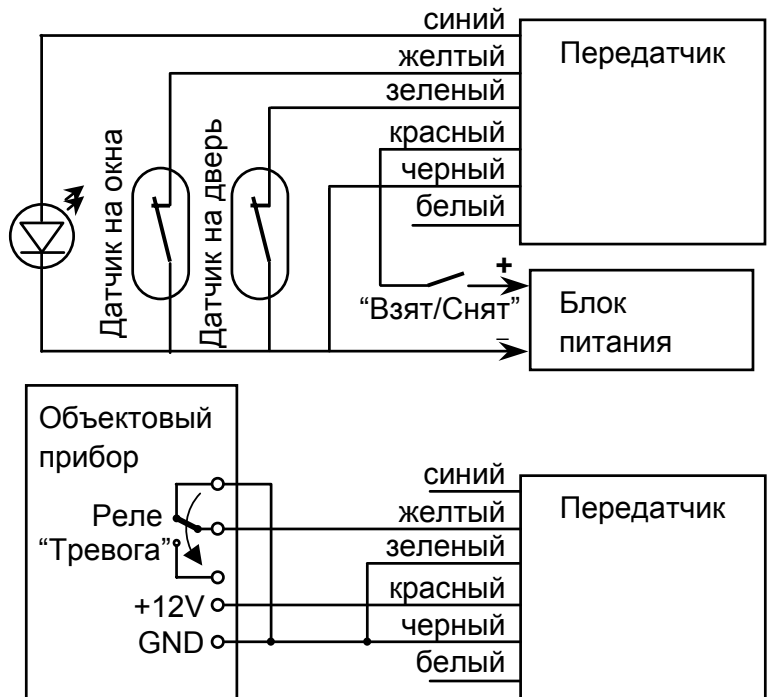
Рис. 3. Примеры монтажа передатчика
