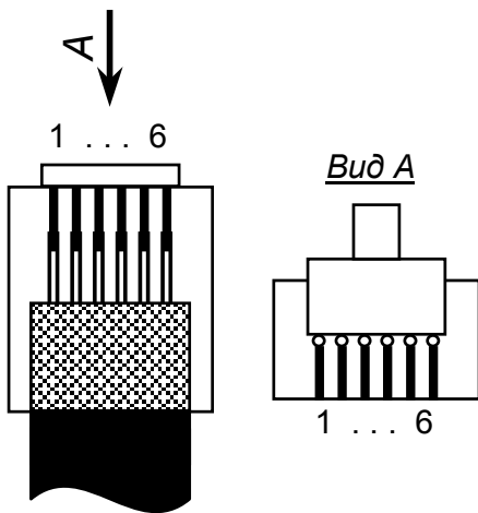
Рис. 2. Разъем
